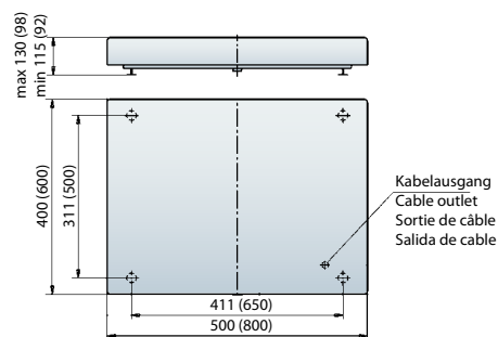
Basamento tipo 150 (350)
